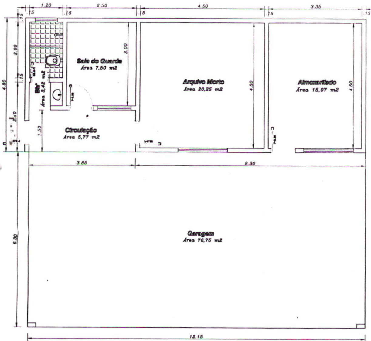
Planta Baixa
